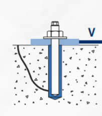
Fallo por desconchamiento
