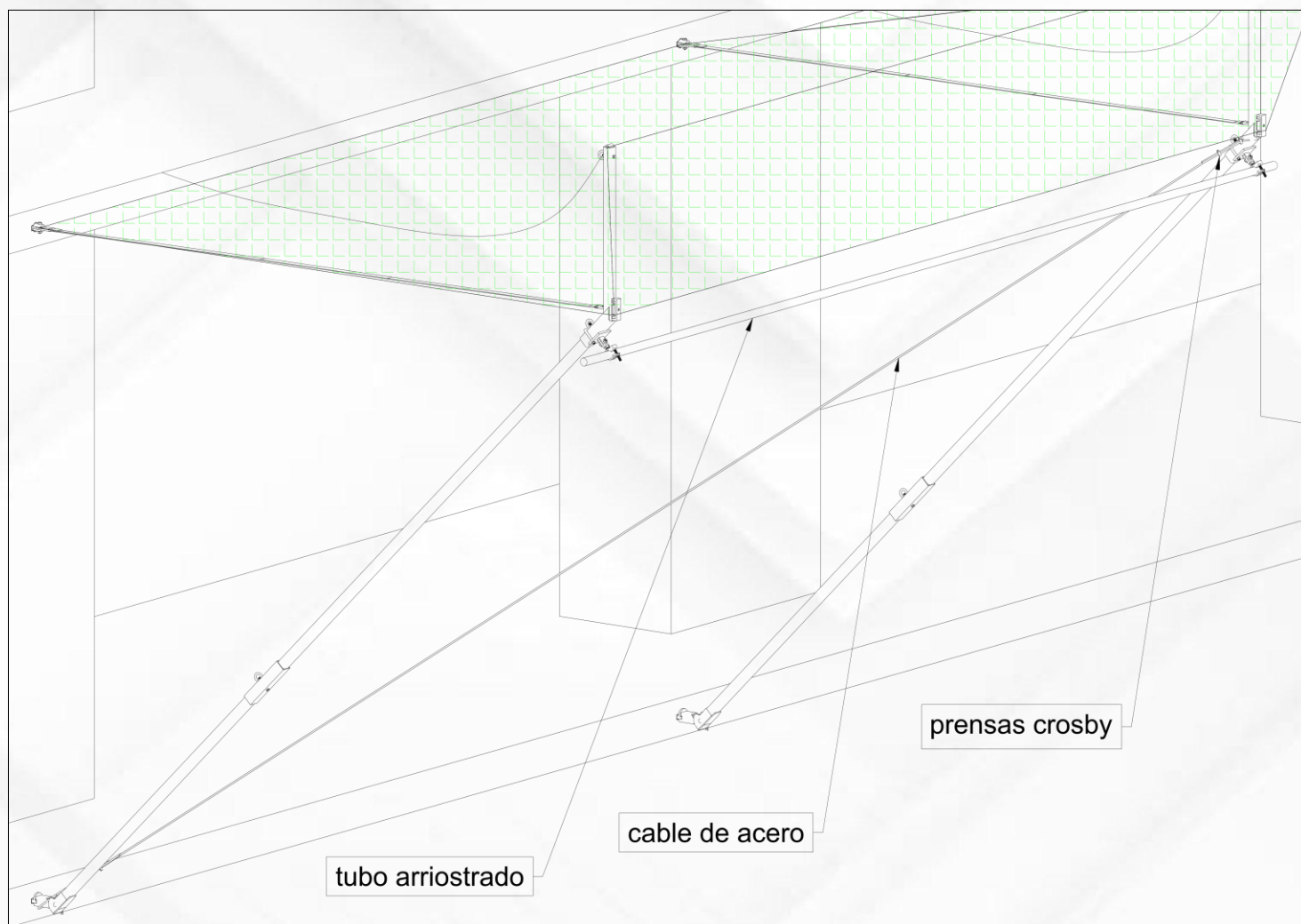
Detalle de arriostrado
