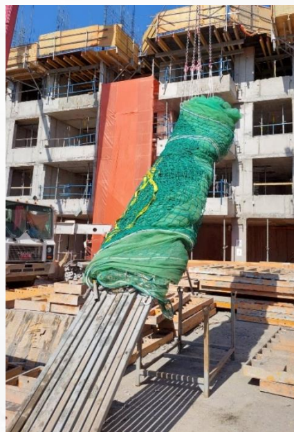
imágenes reales de elevación del sistema de red tipo "T"
