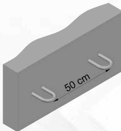
Detalle de vista isométrica de la losa con los omegas instalados.
